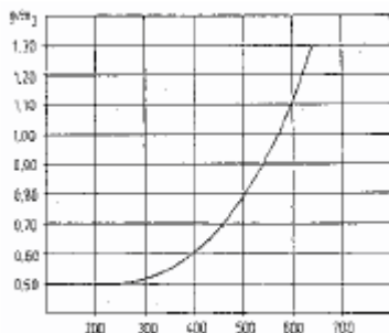
Temperatura de precalentamiento del aire de combustión
